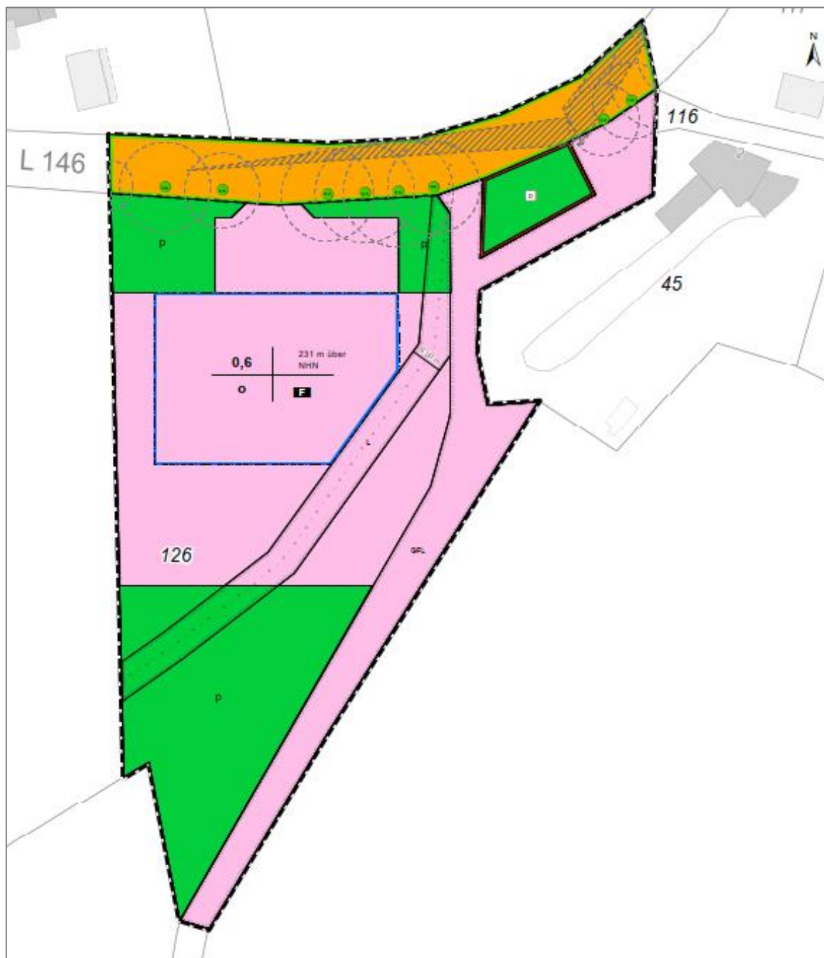
Abbildung 1: Bebauungsplan 112 „Feuerwehrgerätehaus Olpe“ (Ausschnitt ohne Maßstab)
